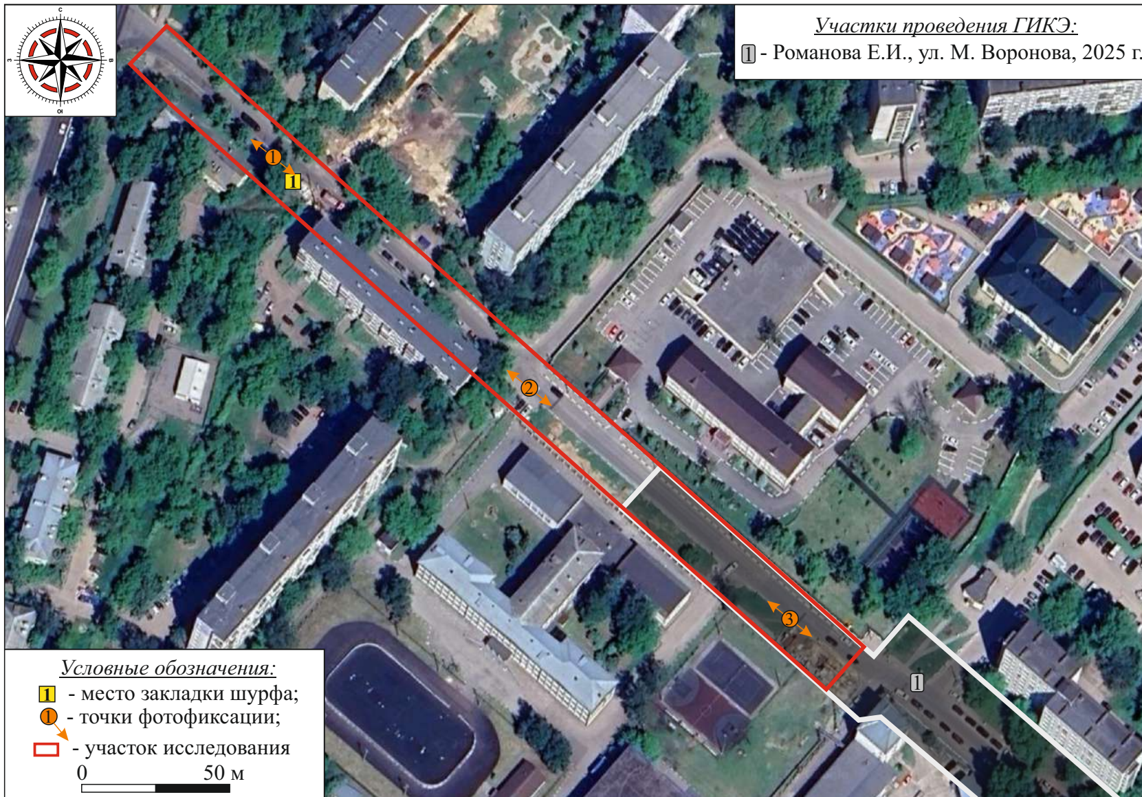
Илл. 8. Нижегородская область, г. Нижний Новгород, Московский р-н, теплотрасса отопления от ТК-314 у д. 18 по ул. Куйбышева - 2026 г. Космоснимок с нанесением участка исследования и расположением шурфа (источник космоснимка: google.ru, дата съемки 2023 г.).
